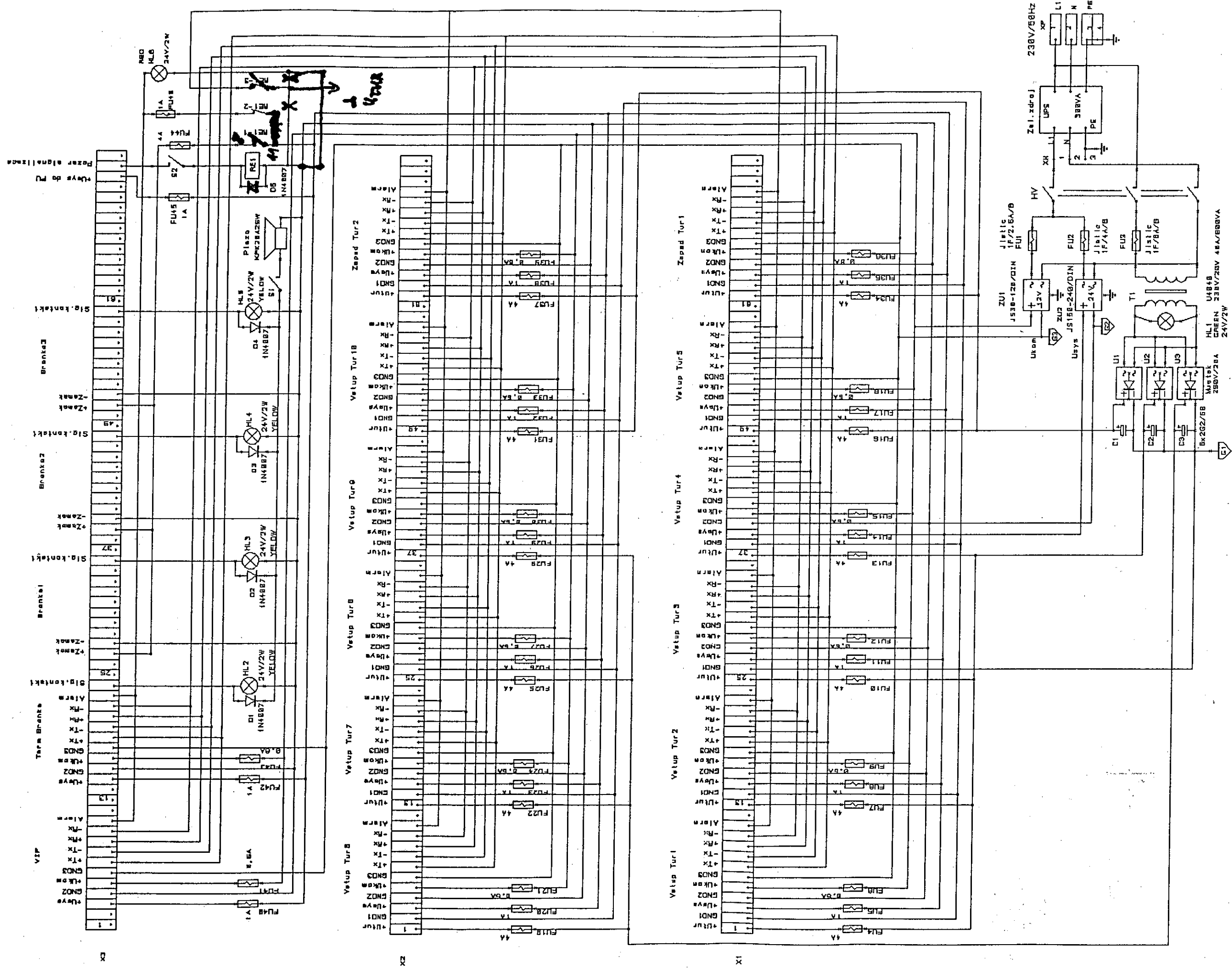
SCHEMA ZAPOJENI ROZVADECE VSTUPNIHO SYSTEMLU - ZIMNI STACION PARDUBICE ID-SYSTEM USTI NAD DRLICI
